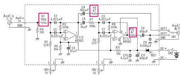
電子回路
